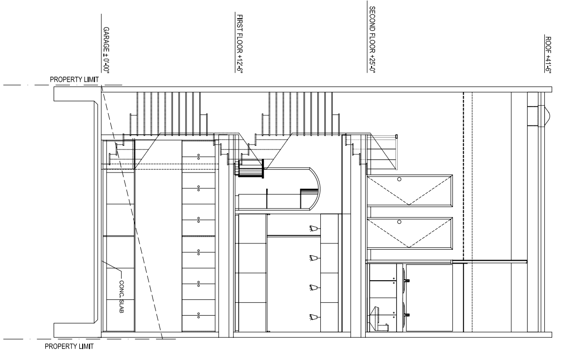
1 SECTION A-A
